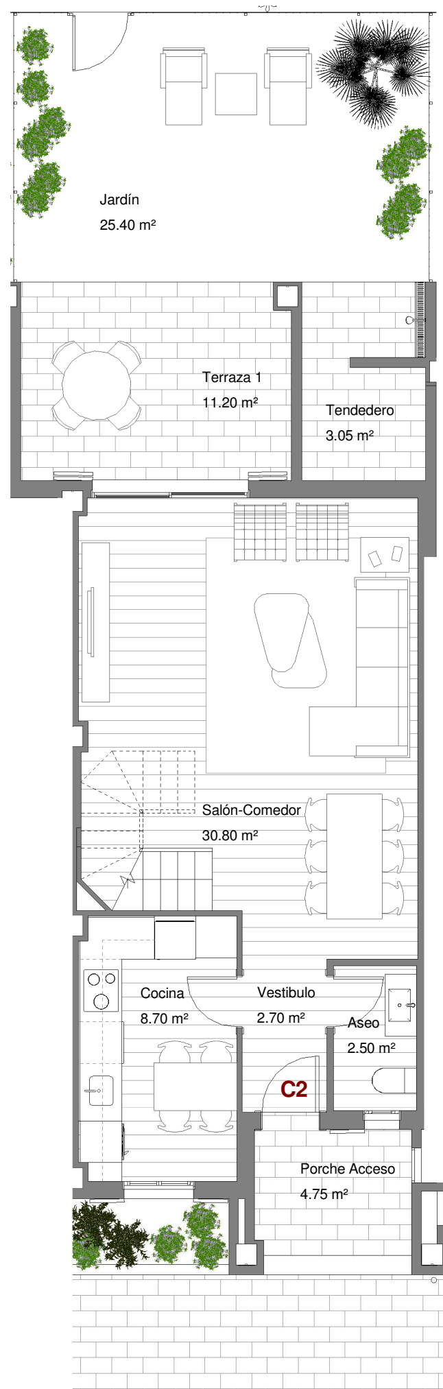
Planta Baja
