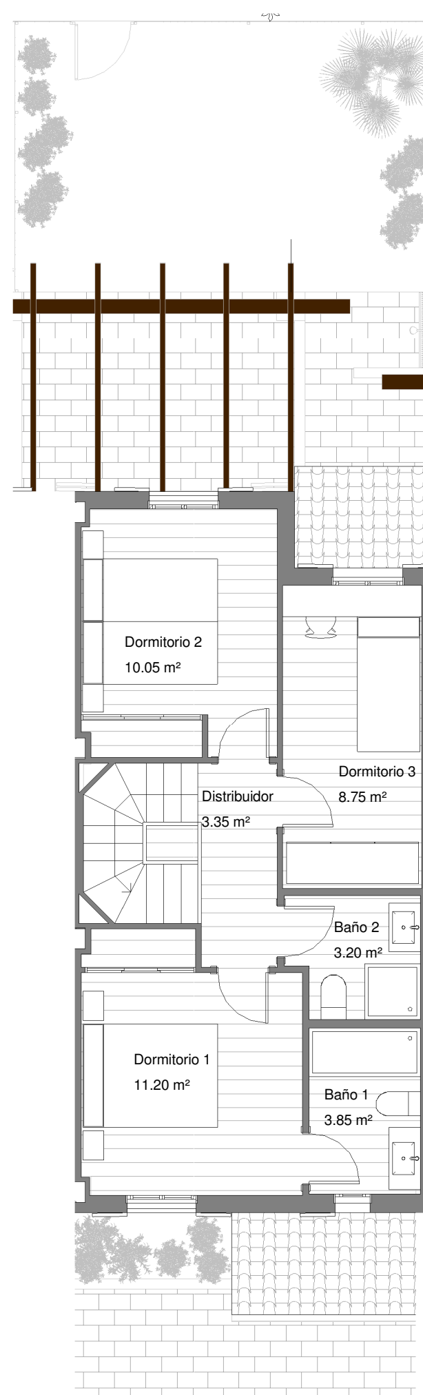
Planta Primera
