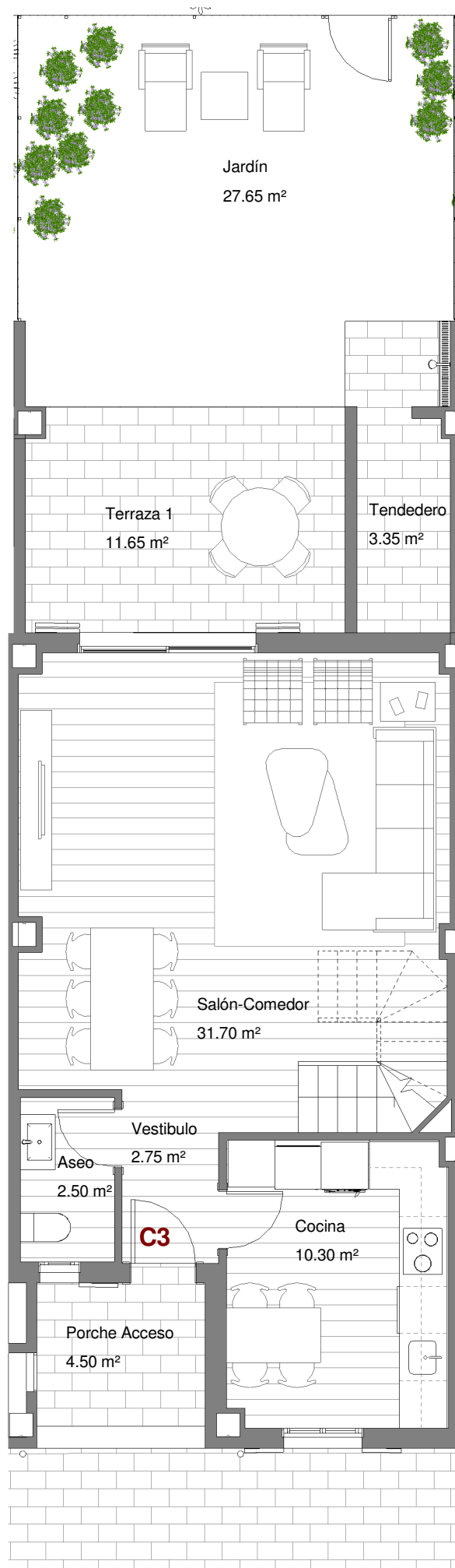
Planta Baja
