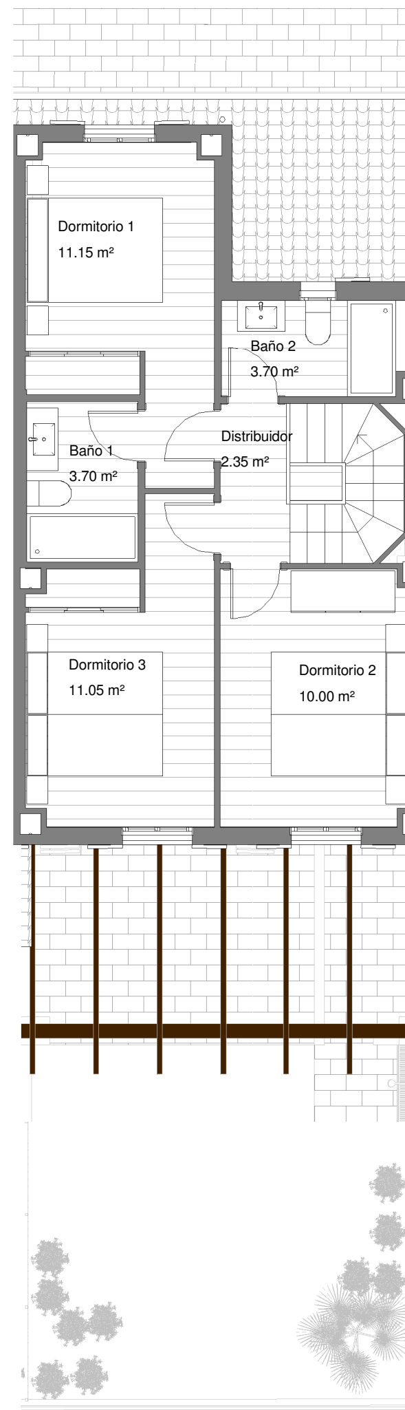
Planta Primera
