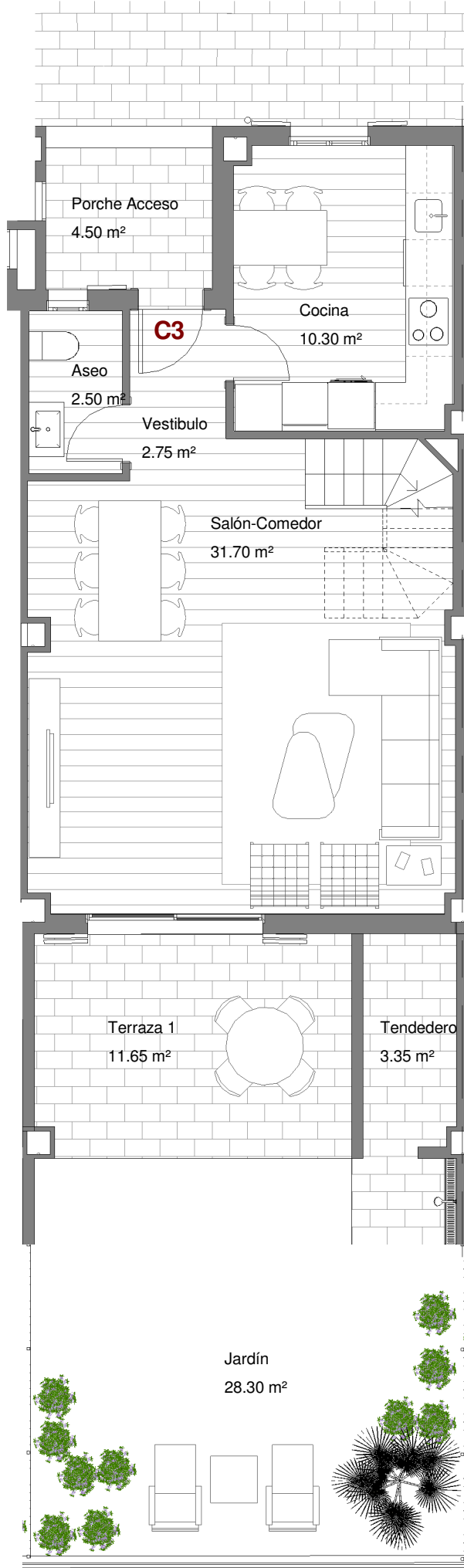
Planta Baja
